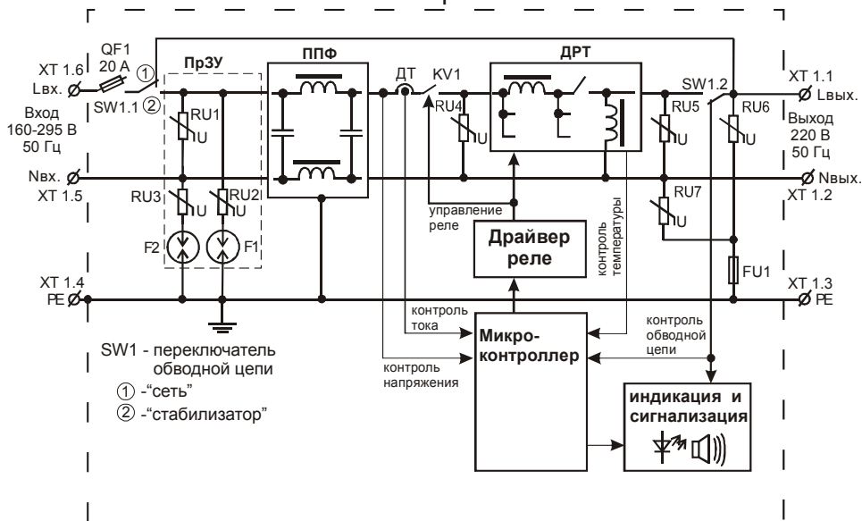
Рисунок 2 – Упрощенная структурная схема стабилизатора
