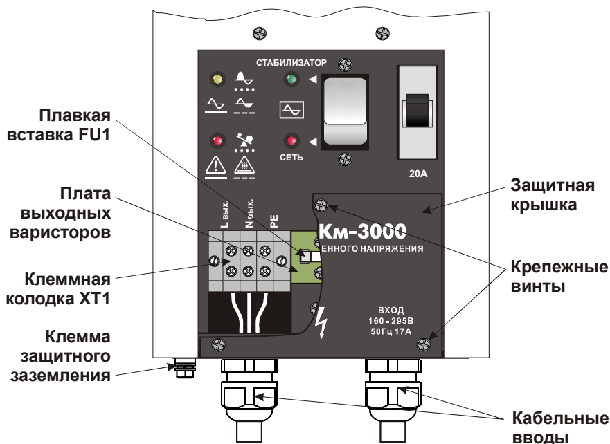
Рисунок 4 – Верхняя панель и органы подключения стабилизатора
