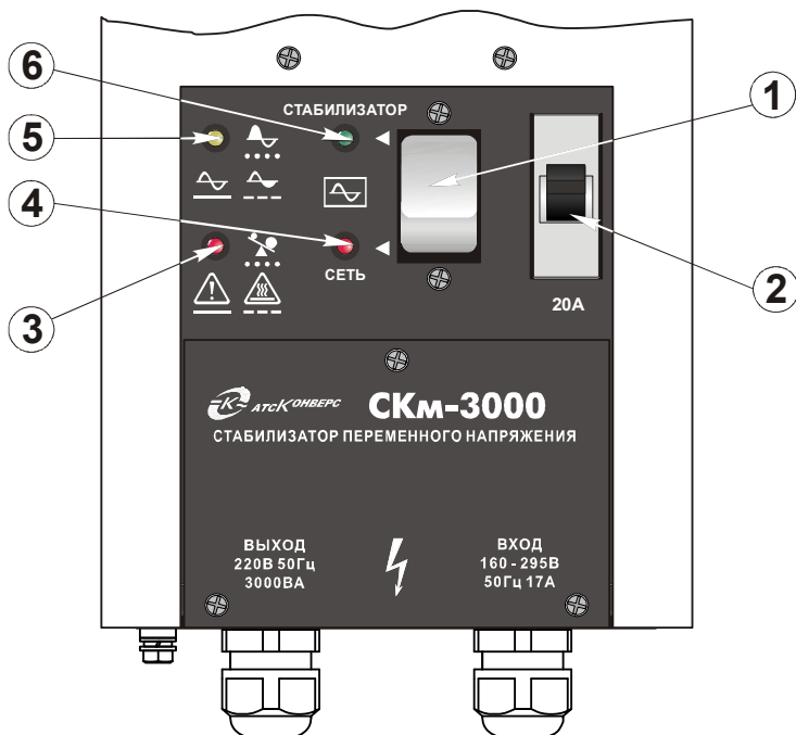
Рисунок 3 – Органы управления и индикации стабилизатора
