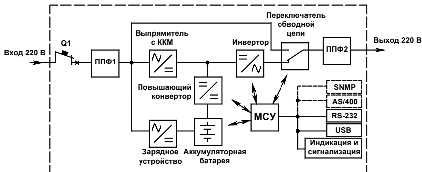
Рисунок 1 - Структурная схема ИБП
