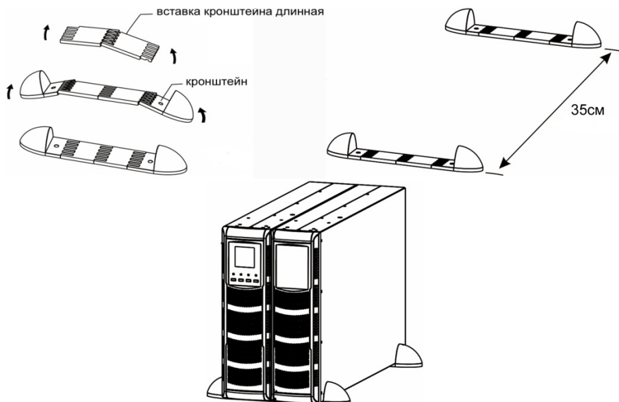
Рисунок 7 – Порядок установки ИБП совместно с БМ в вертикальное напольное (настольное) положение
