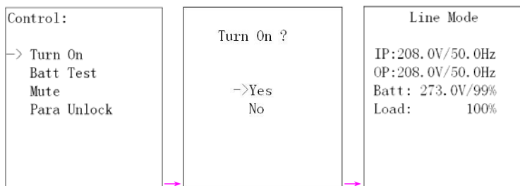
Рисунок 13 – Последовательность включения ИБП
