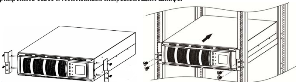
Рисунок 5 – Порядок установки ИБП в стандартный шкаф или стойку для телекоммуникационного оборудования шириной 19 дюймов
